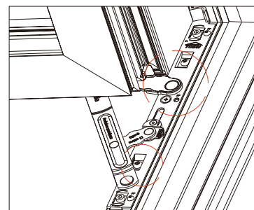
螺钉固定 Screw fixation
