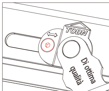
螺钉固定 Screw fixation
